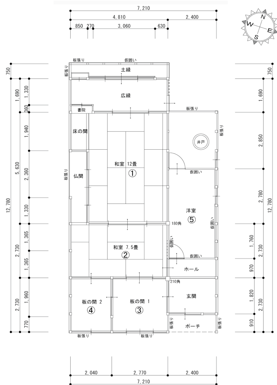
1階平面図
