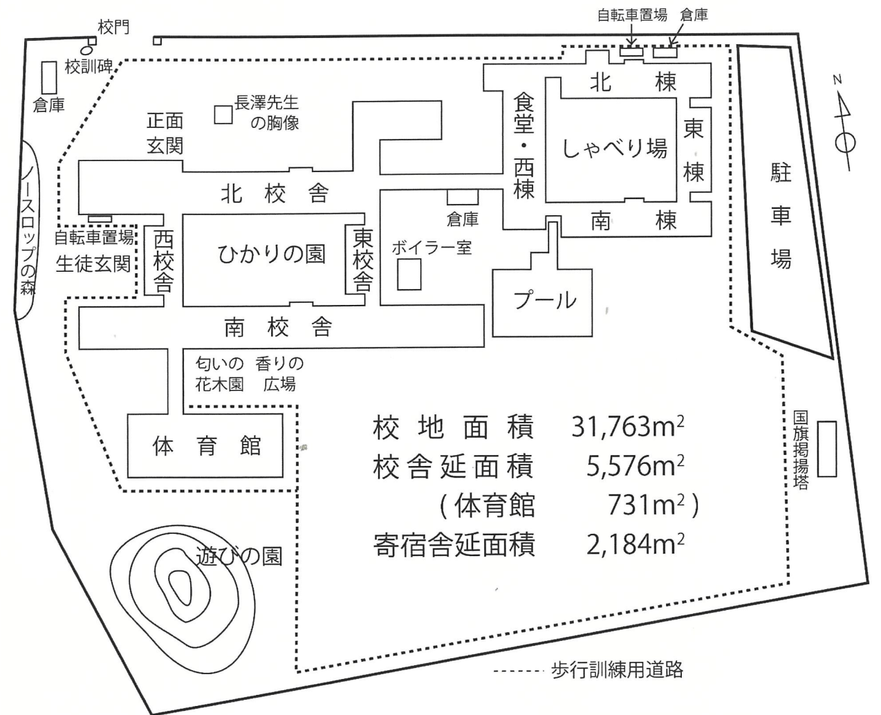
18 校地平面図
