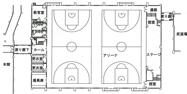
1階平面図
