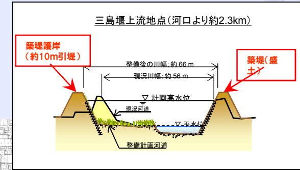
横断図
