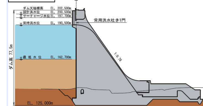
標準断面図
