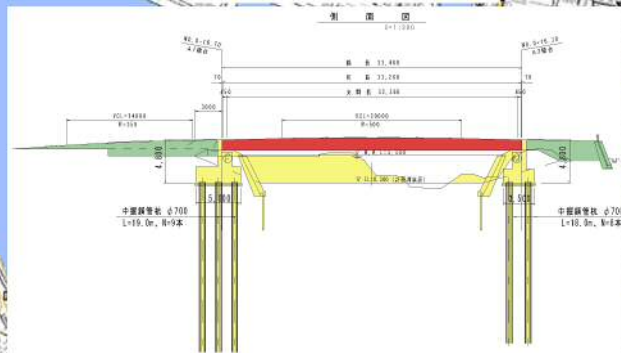
市塔橋(側面図)
